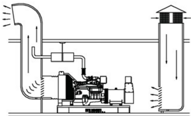
Рис. 4.4. Воздушная вентиляция
