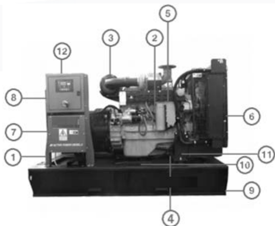
Рисунок 3.1 Типовая конфигурация ДГУ
