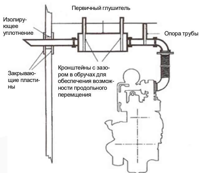
Рис. 7.2. Система выхлопа
