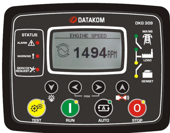
Рис. 15.1. Контроллер DKG D300
